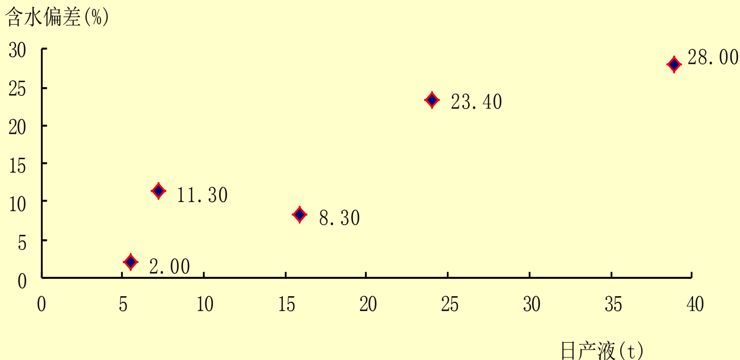
关严生产闸门产生的含水偏差与日产液关系 图1
